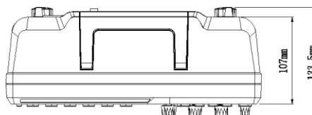
2-Kanal Oszilloskop Draufsicht
