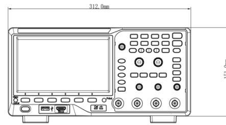
4-Kanal Oszilloskop Frontansicht
