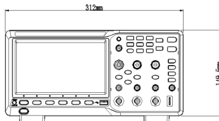
2-Kanal Oszilloskop Frontansicht
